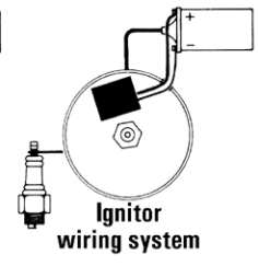
18-5296-2D Display Package 18-5296-2 KIT CONVERSIÓN ELECTRÓNICO Para: Mayoría de Mallory YL o YD 8 cil., rotación normal y contratación.
