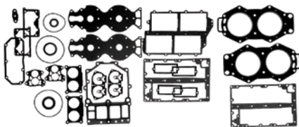
18-4411 JUEGO JUNTAS BLOQUE MOTOR Reemplaza: 6N6-W0001-03-00, 6N6-W0001-A3-00 — CONTIENE —
