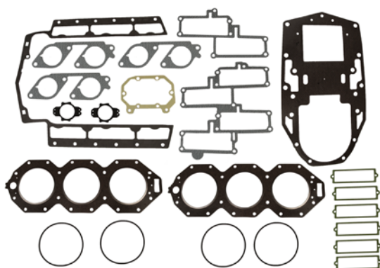
18-4421 KIT JUNTAS MOTOR Reemplaza: 5000400 Para: 90 Ficht FFI, 115 Ficht FFI, 135 Ficht FFI
