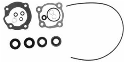
18-2657 KIT RETENES UNIDAD INFERIOR Reemplaza: 396352
