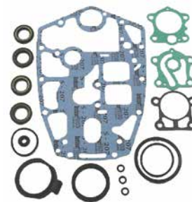
18-2787 KIT RETÉN ALOJAMIENTO ENGRANAJE Reemplaza: 698-W0001-20-00, 698-W0001-C0-00
