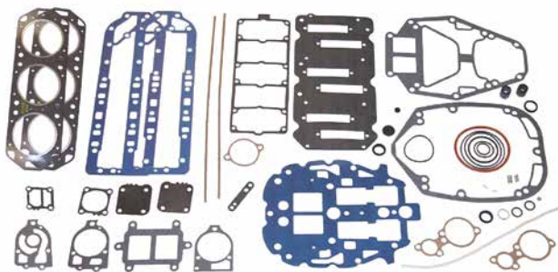
18-4339 JUEGO DE JUNTAS BLOQUE Reemplaza: 27-14697A87 Para: V200EFI y V220 fueraborda
