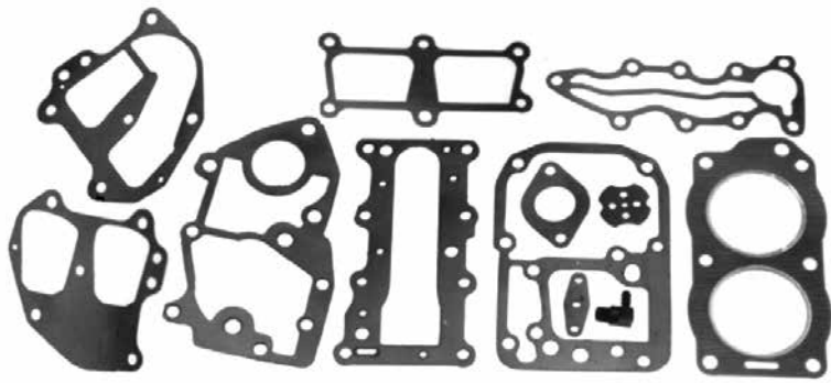
18-4306 KIT JUNTAS MOTOR Reemplaza: 394546
