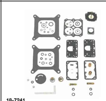
18-7241 KIT CARBURADOR Reemplaza: 3855017 Para: 7.4L GL, 8.2L GL
