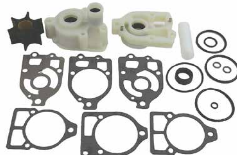
18-3321 KIT BOMBA AGUA Para: #1 Units con enjuague S/N 2495186-2763441
