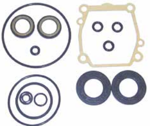
18-8381 KIT RETENES PARTE INFERIOR Reemplaza: 25700-99E00 Para: DF 60(2001 & Sup), DF70(2001 & Sup)
