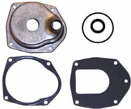
18-3571 KIT ALOJAMIENTO BOMBA Reemplaza: 817275A1 V-6 fueraborda
