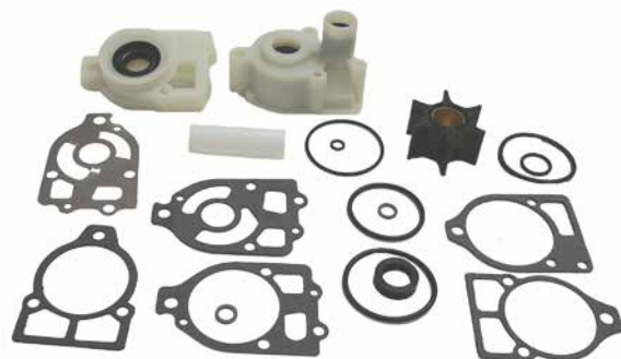
18-3317 KIT BOMBA AGUA Para: #1/R Units sin enjuague S/N 2763442-6854392
