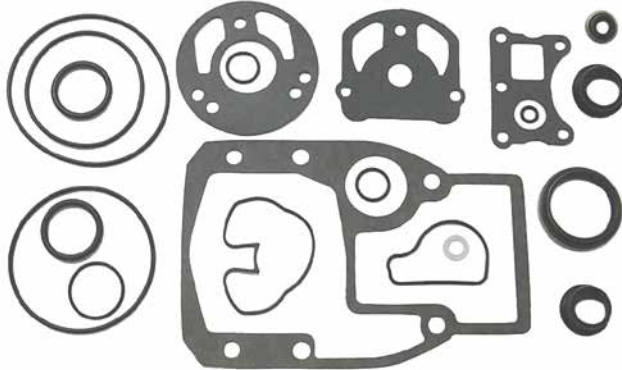
18-2673 KIT RETENES UNIDADES SUPERIOR Reemplaza: 984459, 986364, 987603 Todos Cobra (1986-89)
