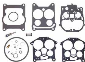
18-7095 KIT CARBURADOR Reemplaza: 983864, 383918
