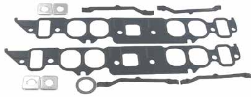
18-0465 JUEGO JUNTAS COLECTOR ADMISIÓN Reemplaza: 27-65184, 27-8M0050224 Para: motores GM 454 CID, 325, 330, 340, 350 HP y 454 Magnums, 7.4L
