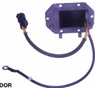
18-5832 REGULADOR/RECTIFICADO Reemplaza: 583266, 583689, 586000, 584424
