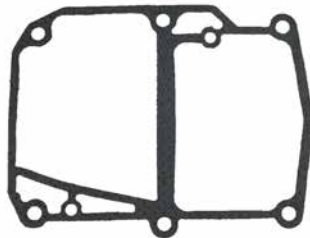
18-99150 JUNTA CÁRTER SUPERIOR Reemplaza: 63V-45113-A1 Para: 9.9(1997-09), 15(1997-09)
