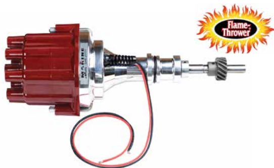
18-5477 DISTRIBUIDOR ELECTRÓNICO Para: motor Ford 302 V-8 Reemplaza tapa/Rotor Kit 18-5266
