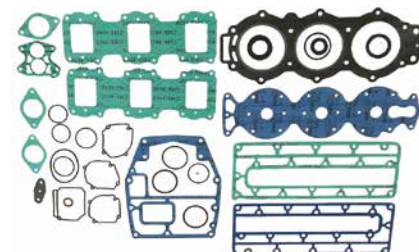
18-4405 JUEGO DE JUNTAS BLOQUE MOTOR Reemplaza: 6H1-W0001-00-00, 6H1-W0001-01-00, 6H1-W0001-A0-00 — CONTIENE —
