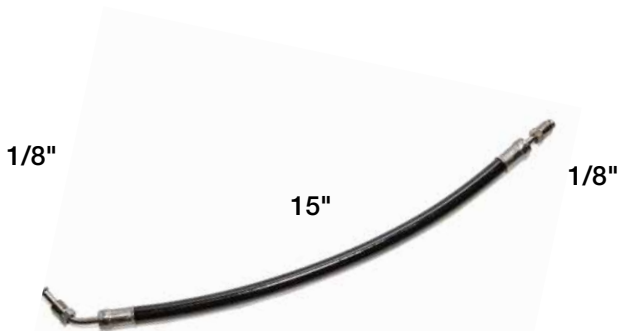
18-2116 LATIGUILLO TRIM Reemplaza: 32-99904, 32-99904Q
