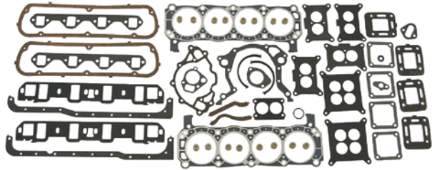
18-4385 Para: Motores Ford 302 (5.0L) CID; 215, 225 & 888 (188 HP) Incluye junta culata 18-3883
