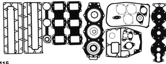
18-4415 JUEGO JUNTAS BLOQUE MOTOR Reemplaza: 688-W0001-00-00, 688-W0001-A0-00
