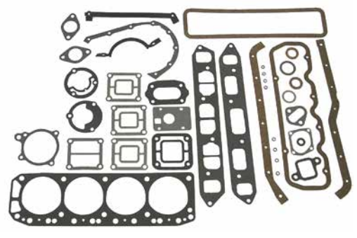
18-4373 JUEGO JUNTAS Para: 110, 120 HP y 2.5L (1965-86)
