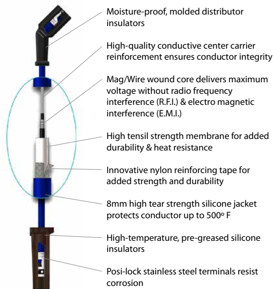
OMC MARINE APLICACIÓN CABLES ENCENDIDO
