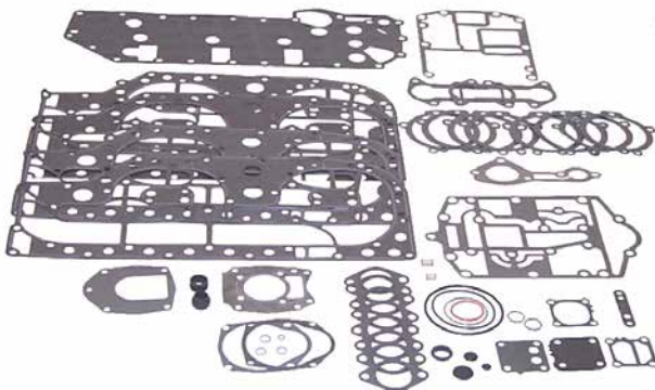
18-4340 JUEGO DE JUNTAS DE BLOQUE Reemplaza: 27-13461A99, 27-13461A90, 27-13461A89, 27-13461A88 Para: 80 Jet, 100HP, 115HP, and 125HP 4 cil Fueraborda
