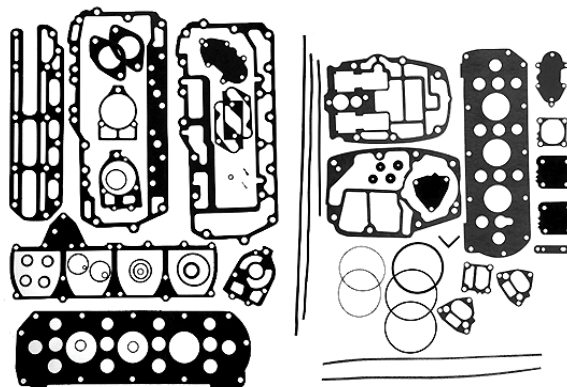
*18-4354 JUEGO DE JUNTAS BLOQUE Reemplaza: 27-73645A87, 27-73645A76, 27-73645A32
