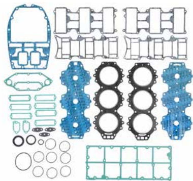
18-4400 JUEGO DE JUNTAS BLOQUE DE MOTOR Reemplaza: 61A-W0001-01-00, 61A-W0001-A1-00 — CONTIENE —
