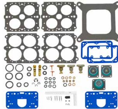
18-7751 KIT CARBURADOR
