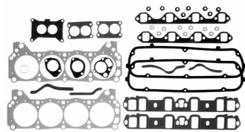
18-4391 JUEGO JUNTAS COLECTOR ADMISIÓN Reemplaza: 27-64763A2 Para: Motores Ford 351 CID; 233 HP S/N 4173000-4500860, 5.8L Incluye junta culata 18-3883
