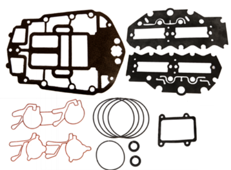
18-4402 KIT JUNTAS MOTOR Reemplaza: 437779, 439559 Para: 90 V4 60 grados (1995-00), 115 V4 60 grados (1995-00)
