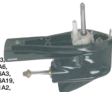
18-2452 UNIDAD SUPERIOR COMPLETA Reemplaza: 1547-9412A22, 1547-5523A67, 1547-8265A17, 1547-9412A36 Para: Alpha I 1.84:1/1.81:1
