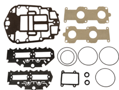
18-4406 KIT JUNTAS MOTOR Reemplaza: 437155 Para: 150 60 grados (1991-00), 175 60 grados (1991-00)
