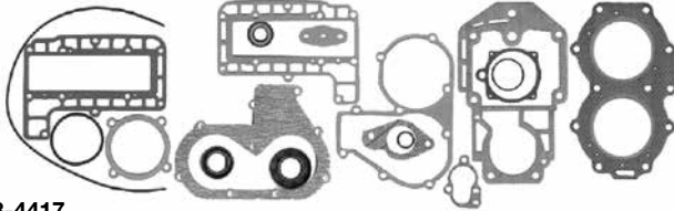
18-4417 JUEGO JUNTAS BLOQUE MOTOR Reemplaza: 695-W0001-01-00, 695-W0001-02-00, 695-W0001-A2-00
