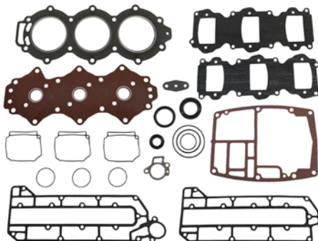
18-99176 JUEGO JUNTAS BLOQUE MOTOR Reemplaza: 6H3-W0001-02 Para: 60(2001-05), 70(1994-09), C70(2000-01), P60(1994-99)
