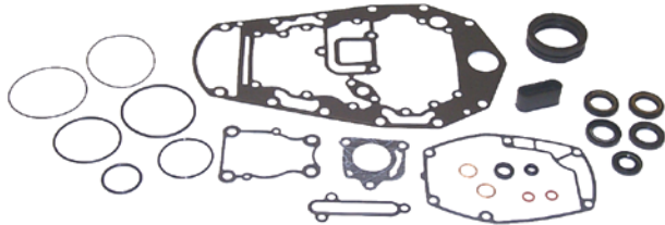
18-0020 KIT RETENES ALOJAMIENTO ENGRANAJES Reemplaza: 67C-W0001-21-00 Para: T25 (2001-02) / F30 (2002) F40 (2002) 3 cil modelo
