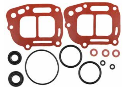
18-74610 KIT SELLADO UNIDAD INFERIOR Reemplaza: 398-87321-0 Para: 18 & 15 (1997-08); 9.9 (1997-04)
