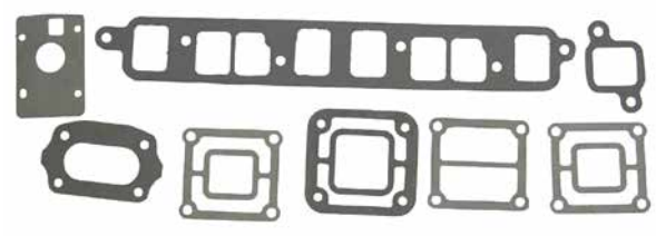
18-4371 JUEGO JUNTAS COLECTOR ESCAPE Para: 140 HP y 3.0L (1973-84)
