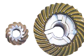
18-2310 JUEGO DE ENGRANAJES AVANCE Reemplaza: 397627 Incluye: engranaje avance y piñón
