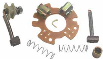
18-6250 KIT REPARACIÓN MOTOR DE ARRANQUE Prestolite 2 Escobillas
