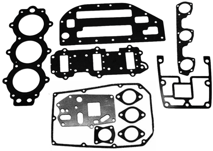
18-4321 KIT JUNTAS MOTOR Reemplaza: 398047, 438904
