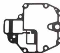
18-99027 JUNTA CÁRTER Reemplaza: 68T-13475-00 Para: F6(2001-08), F8(2001-10), F9.9(2007, 2010), T8(2001-10), T9.9(2007-10)
