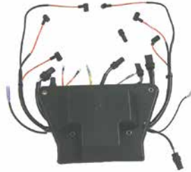
18-5893 CAJA ENCENDIDO Reemplaza: 586667, 584037, 586217, 583476 Para: V-4 & V-8 6700 rpm limite
