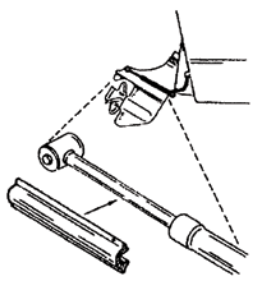
18-9098 BLOQUEADOR COLAS Reemplaza: 174448 Juego de 2 Para todos los modelos SX hasta 2006
