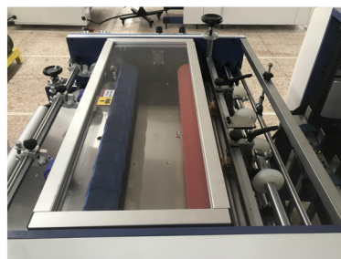
Stacker automático
