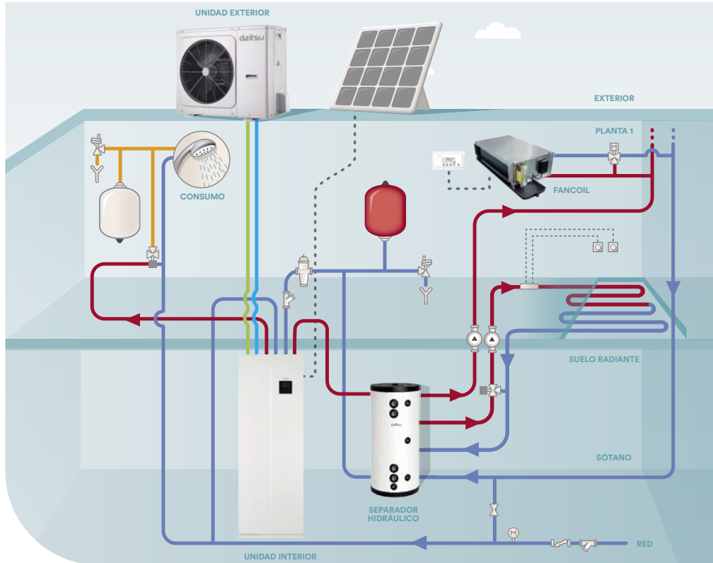
Aplicación Space II con depósito de ACS, suelo radiante y fancoils.
