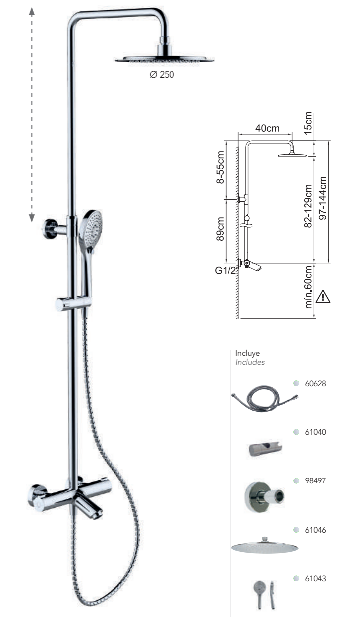
Conjunto de baño-ducha termostática con barra extensible con soporte articulado deslizante. Thermostatic bath-shower set with extendable bar with sliding articulated support.
