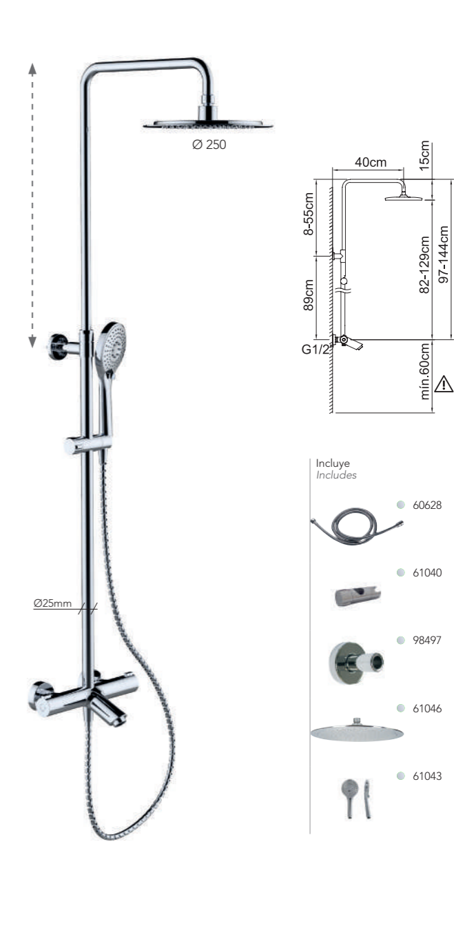
Conjunto de baño-ducha termostática con barra extensible con soporte articulado deslizante. Thermostatic bath-shower set with extendable bar with sliding articulated support.
