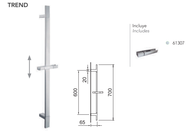
Barra de ducha Trend 30x10x700mm. Trend shower bar 30x10x700mm.
