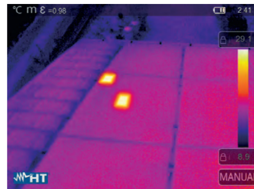
Derecha: Termografía de un panel fotovoltaico con dos puntos calientes captados con THT300.
