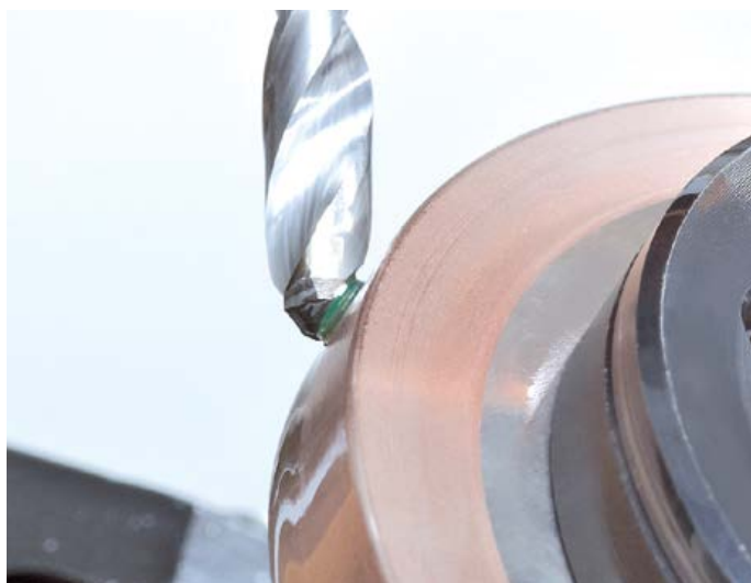
/// EROSIÓN DE BROCAS de una punta helicoidal de PCD
