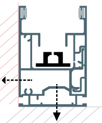
GUÍA ARV COULISSE ARV (HAUTE RÉSISTANCE AU VENT) HWR guide rail (high wind resistance)
