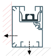
GUÍA ÚNICA COULISSE UNIQUE Única guide rail
