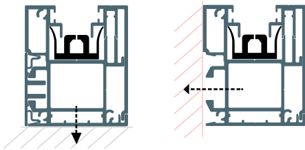
GUÍA SISTEMA TENSIONADO COULISSE SYSTÈME TENDU Tension guide rail system
