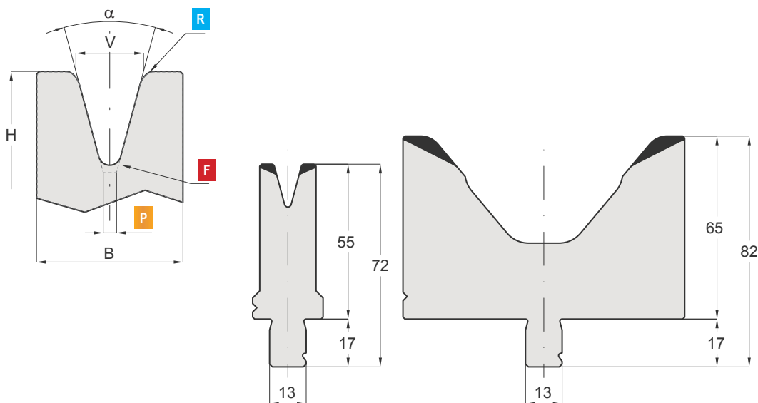
TEMPRA AD INDUZIONE 52-55 HRC INDUCTION HARDENED 52-55 HRC
