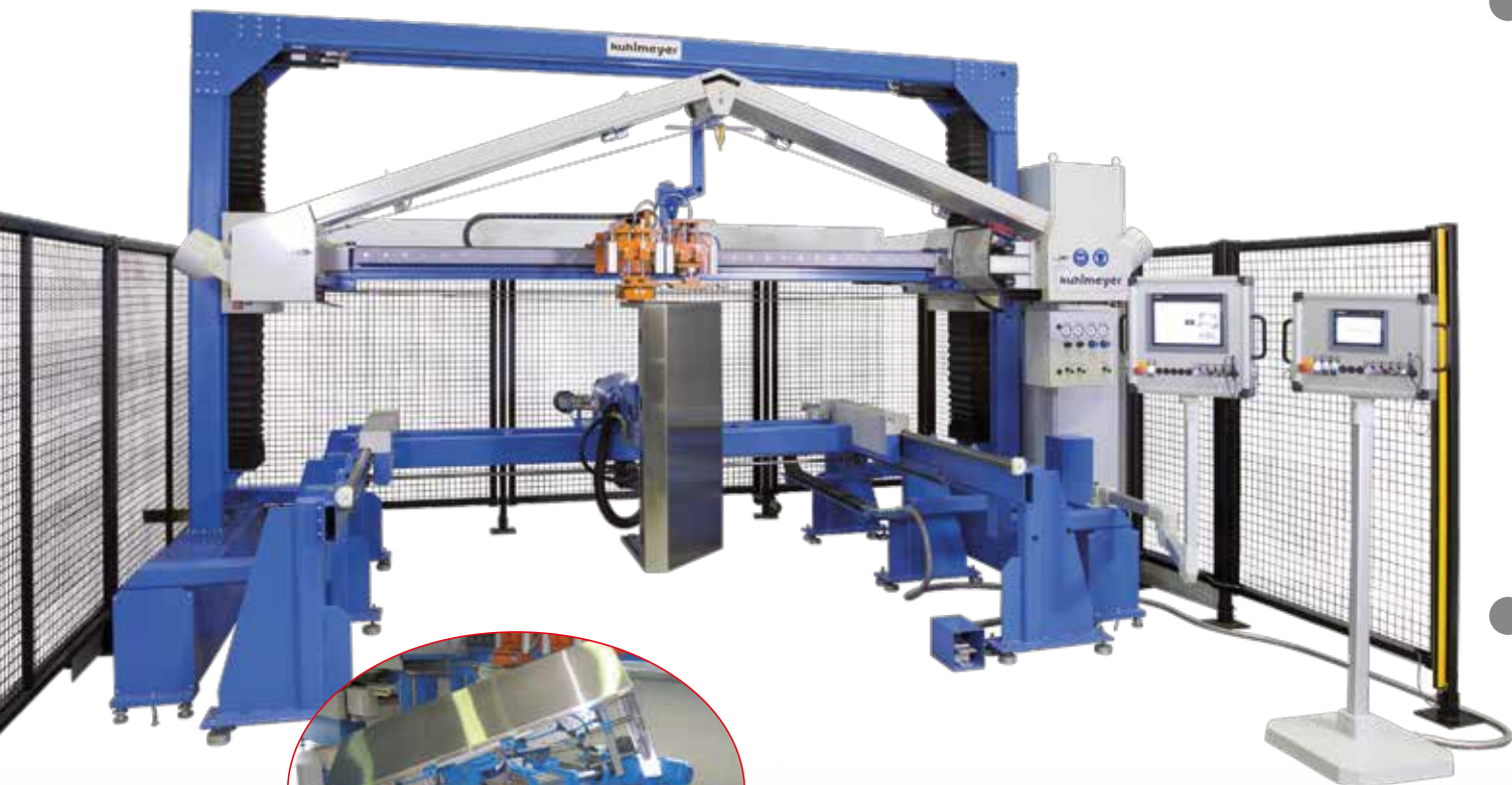
Desbarbadora pulidora Kuhlmeier modelo PZM automática, para piezas de grandes dimensiones.
