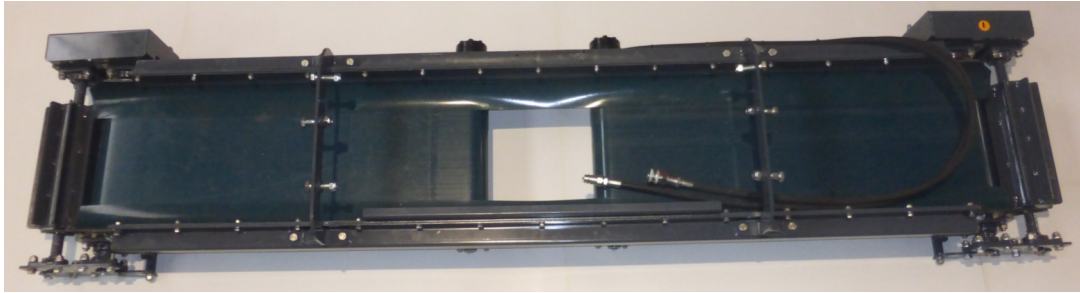
Doble cinta fija hidráulica con rodillos lanzadores plegables - Con 2 caídas dcha./izq. - Con 3 caídas dcha./izq./centro
