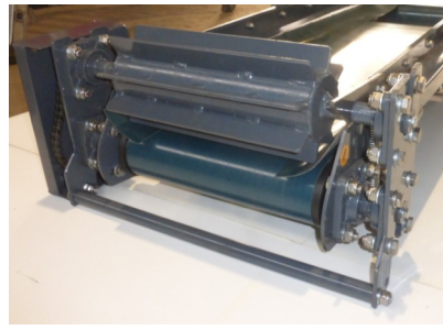
Rodillo lanzador plegable
