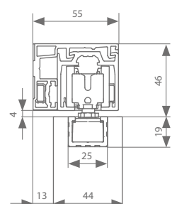
Fijación vista a pared 44 mm
