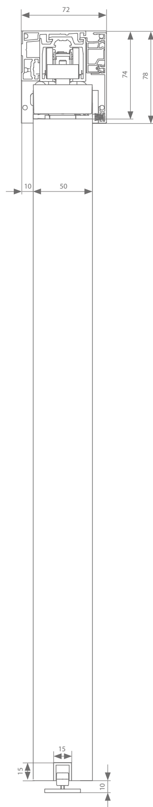
Fijación vista a pared 50 mm
