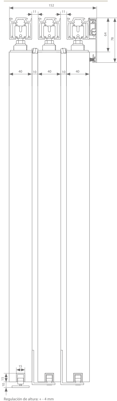
Paralelo fijación vista a techo 1
