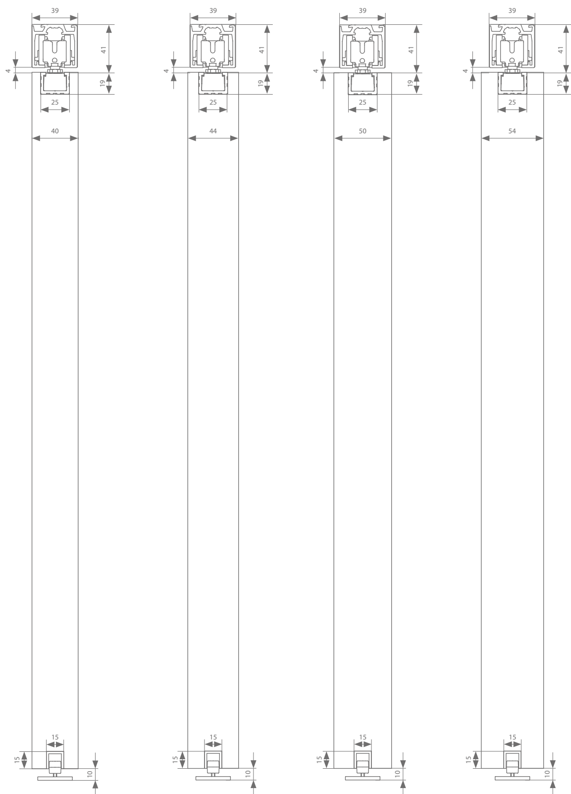
Fijación vista a techo 40 mm Fijación vista a techo 44 mm Fijación vista a techo 50 mm Fijación vista a techo 54 mm
