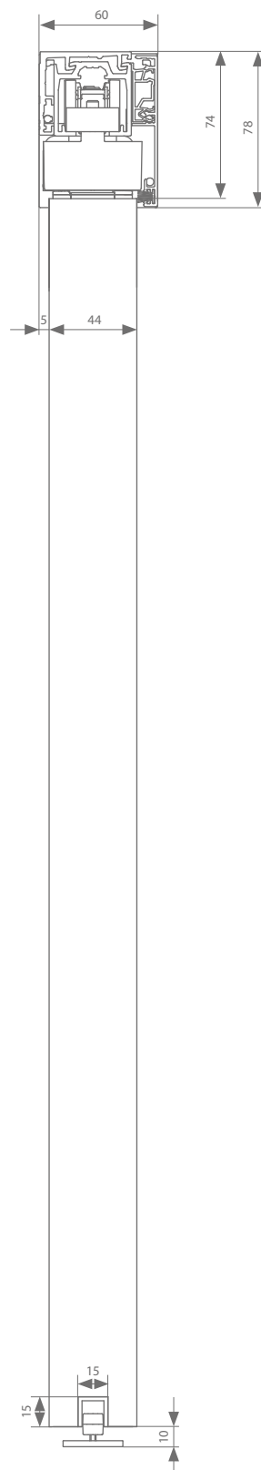
Fijación vista a pared 44 mm
