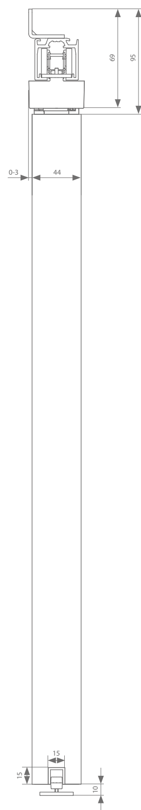
Fijación vista a pared 44 mm
