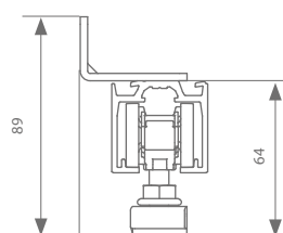
Fijación vista a pared 50 mm
