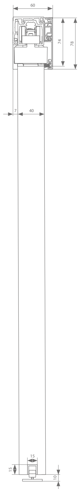
Fijación vista a pared 40 mm
