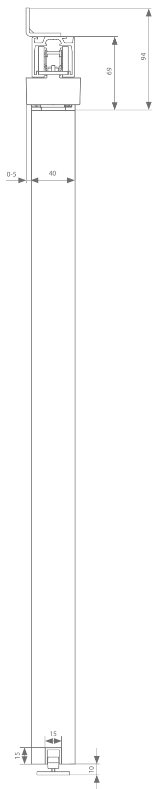
Fijación vista a pared 40 mm
