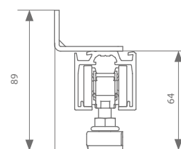
Fijación vista a pared 54 mm
