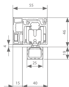
Fijación vista a pared 40 mm
