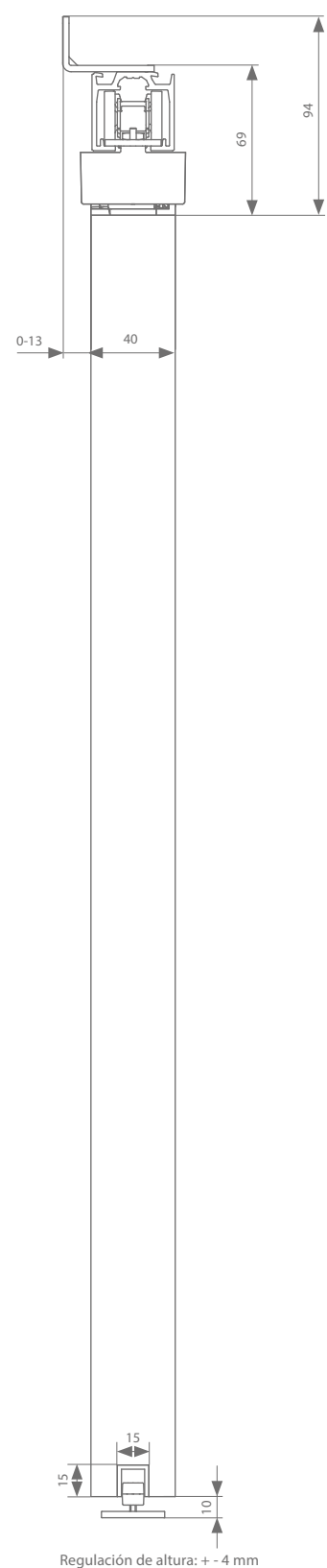
Fijación vista a pared 40 mm
