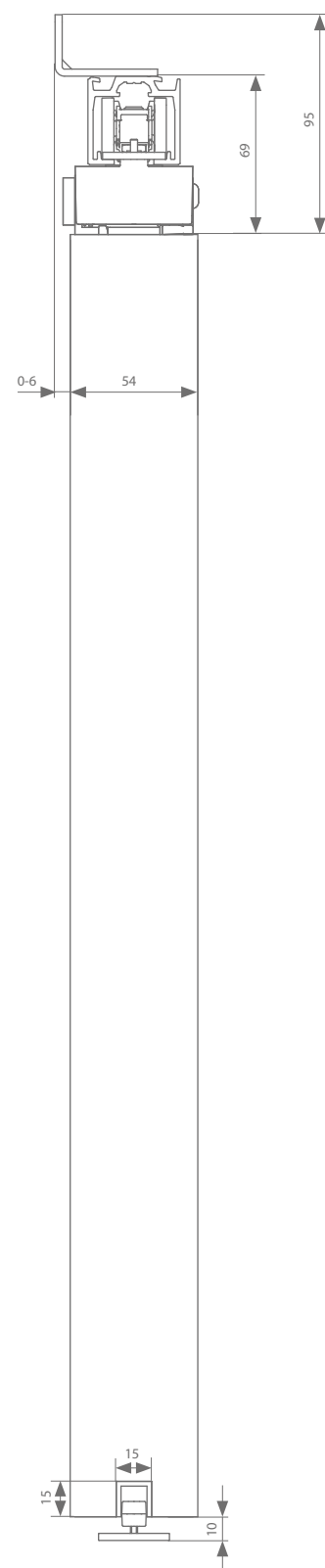
Fijación vista a pared 54 mm
