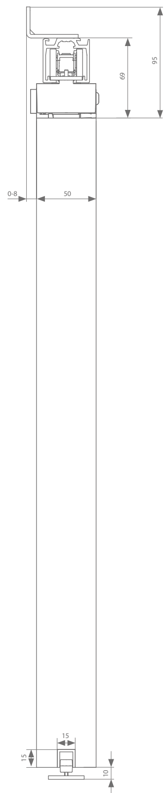
Fijación vista a pared 50 mm
