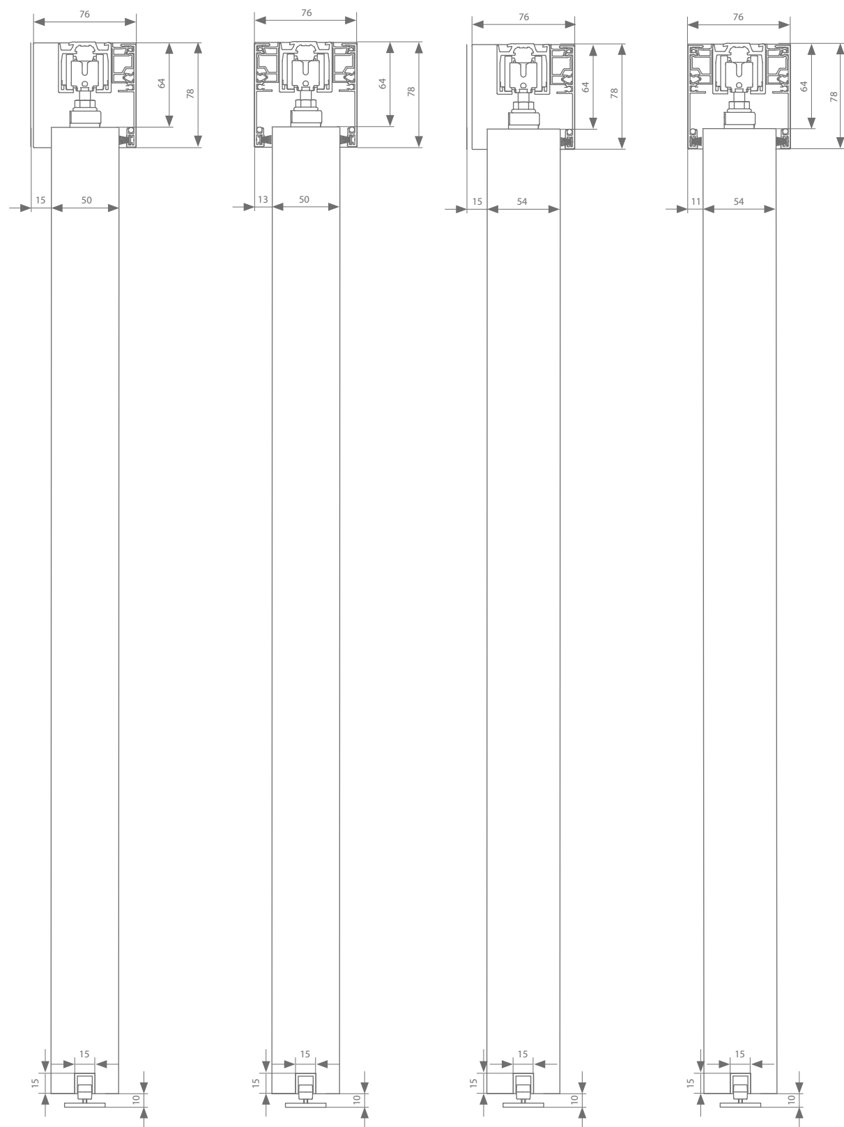
Fijación vista a techo 50 mm
