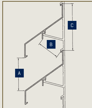
A. Distancia visual entre 2 lamas B. Abertura más estrecha entre 2 lamas C. Paso de la lama
