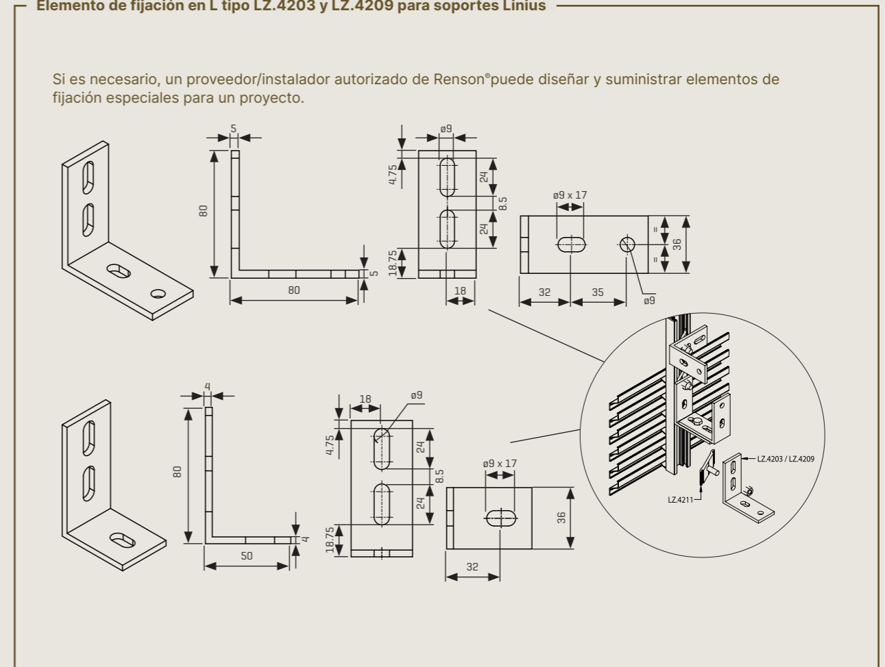
Elemento de fijación en L tipo LZ.4203 y LZ.4209 para soportes Linius
