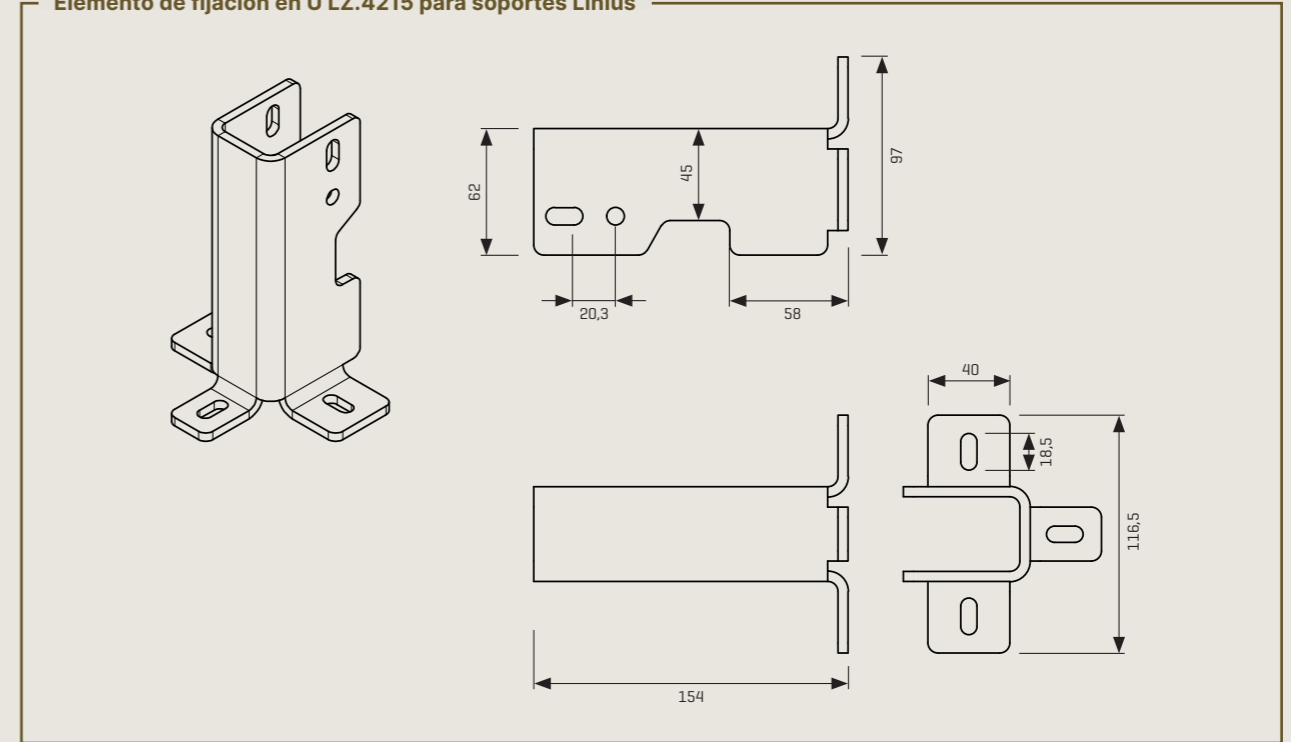
Elemento de fijación en U LZ.4215 para soportes Linius
