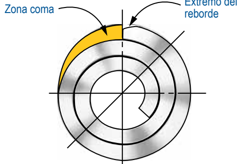
El extremo del reborde está diseñado para esconderse dentro del diámetro del orificio.
