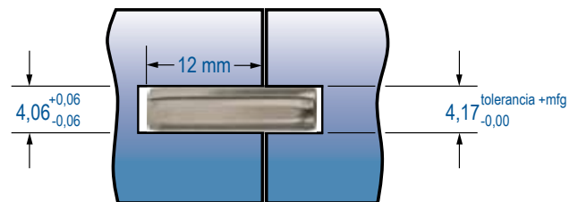
Tamaño recomendado del orificio para ajuste con holgura con CLDP 4 x 20 LBK
