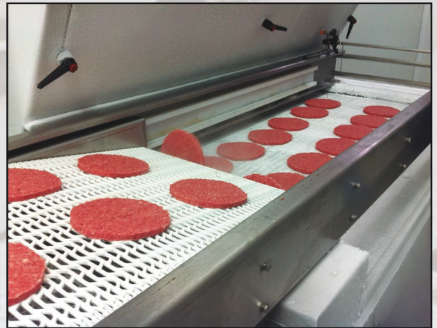
Transportador retráctil
