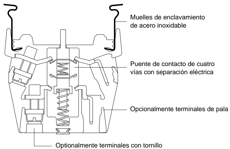
Principio de diseño de los elementos de contacto EF
