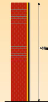
Si la altura es mayor de 18 m, se debe proteger la espuma con un enfoscado de cemento de 1,5 cm
