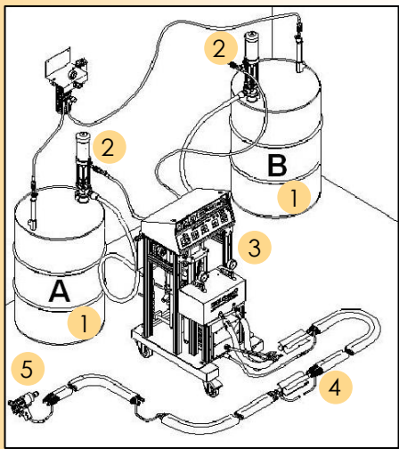
Esquema de una máquina para proyectar espuma de poliuretano:
