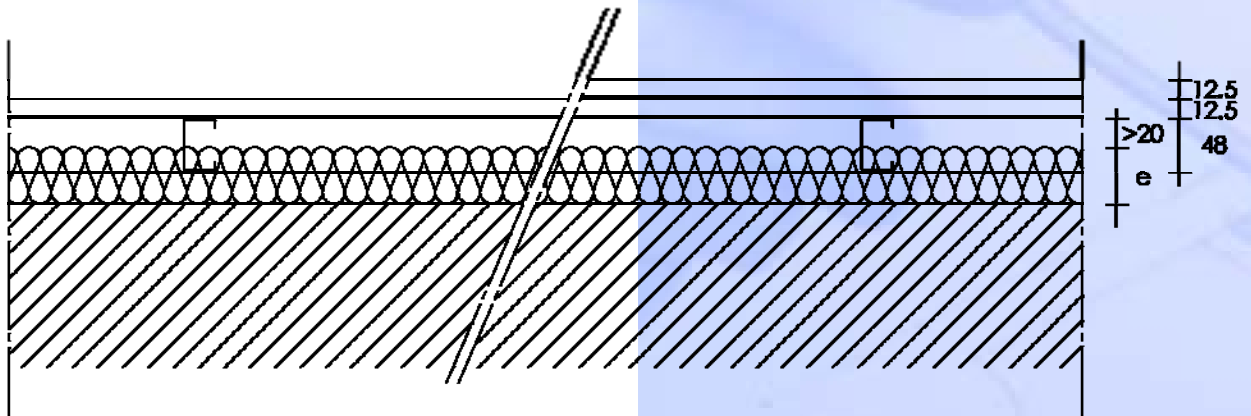
Solución constructiva en la que, al no haber suficiente espacio, la espuma de poliuretano ha de ocupar parte del espacio entre la estructura del trasdosado de yeso laminado.
