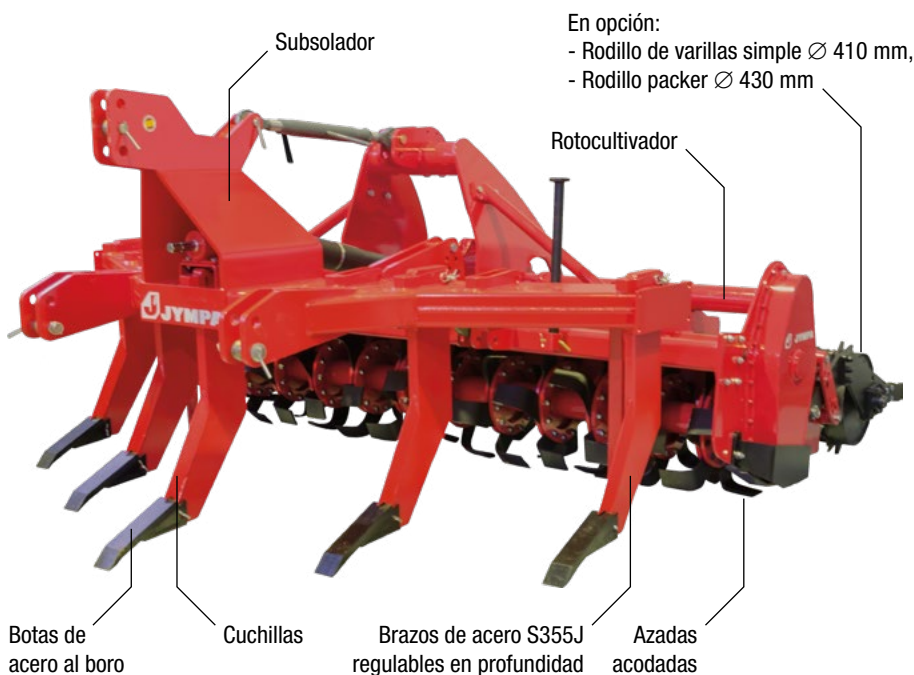
Modelo DUPLA-3000-R con rodillo de varillas simple \varnothing 410 mm
