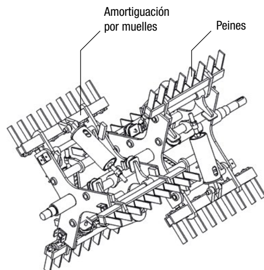
Rotor MYMERTIA
