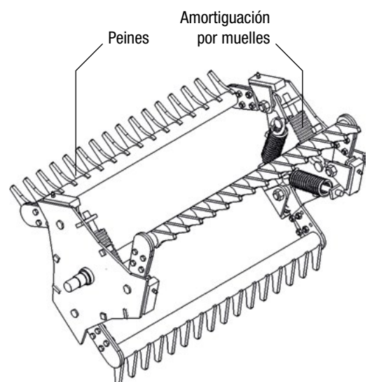
Rotor MYMESIA
