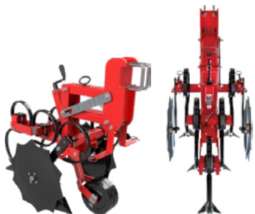
Con disco de protección de la planta
