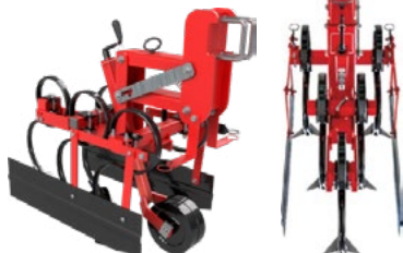
Con chapa de protección de la planta
